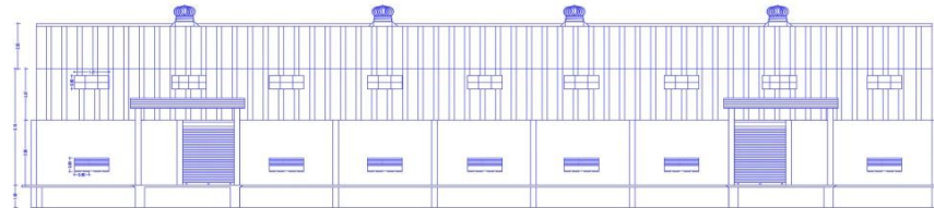
ELEVATION
